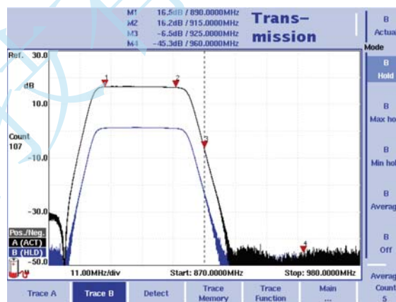
利用9150跟踪发生器选件测量放大器特性
